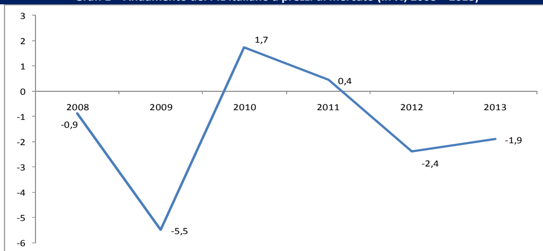
Graf. 1 – Andamento del PIL italiano a prezzi di mercato (In %; 2008 – 2013)
